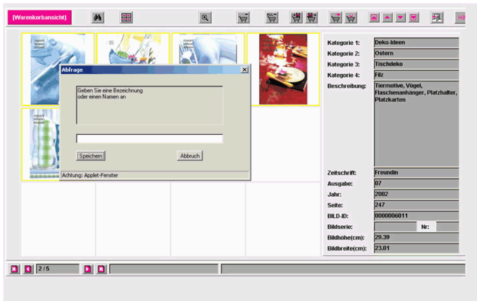
Warenkorbansicht
