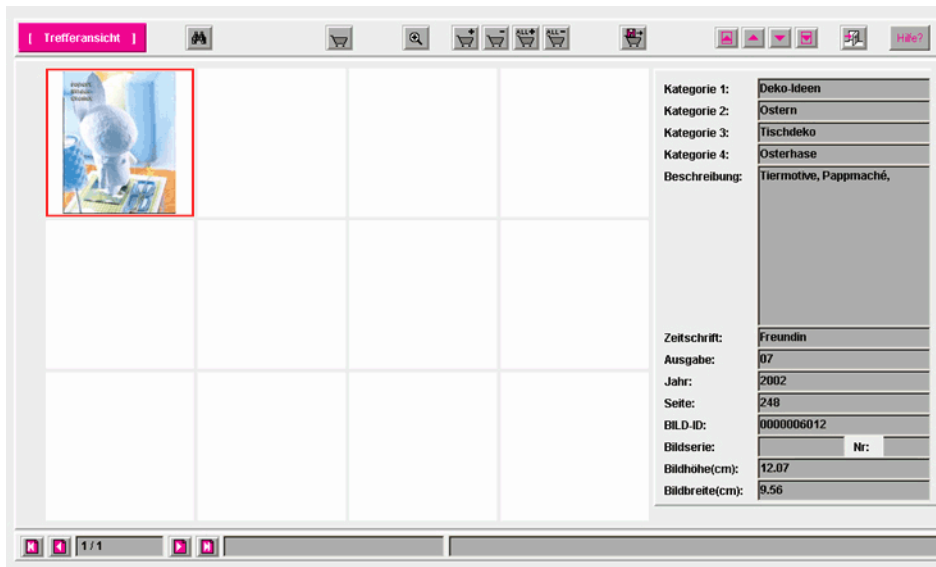
Trefferansicht
