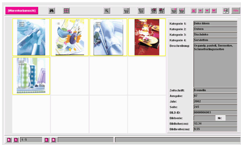
Warenkorbansicht
