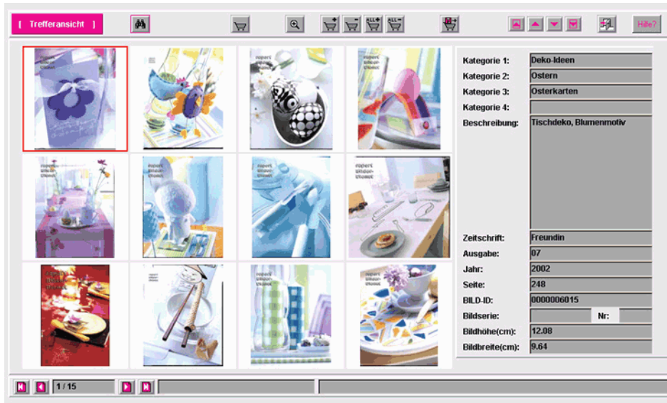
Trefferansicht
